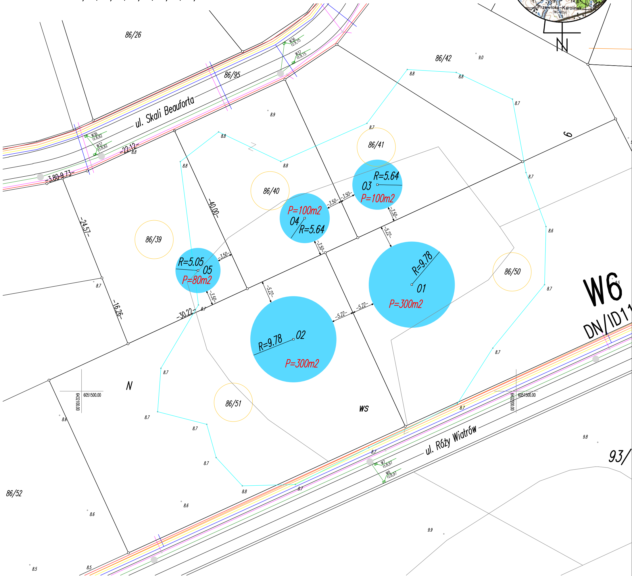
WYKAZ WSPÓLRZĘDNYCH POŁOŻENIA PROJEKTOWANYCH OCZEK WODNYCH układ współrzędnych odniesienia "2000"
